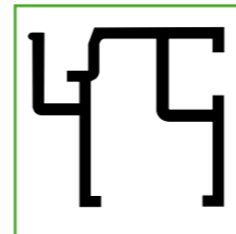
2. Bodenprofil Front und Rückwand Floor profile section of front and back wall Profilé à fixer au sol de la paroi avant et arrière Bodemprofil voor- en achterwand
